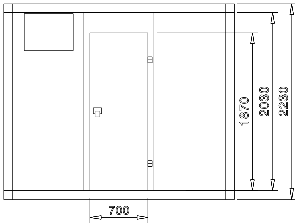
Zij aanzicht
